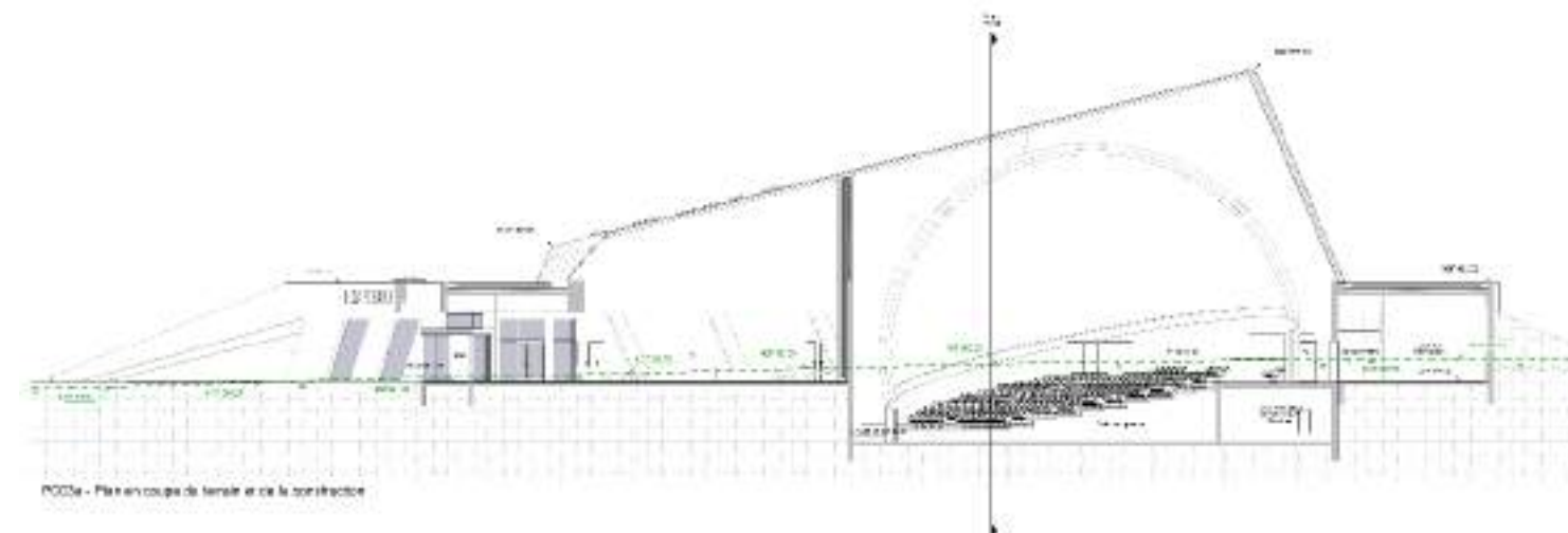
Figure 18 : Coupe du projet de planétarium retenu – source : permis de construire
