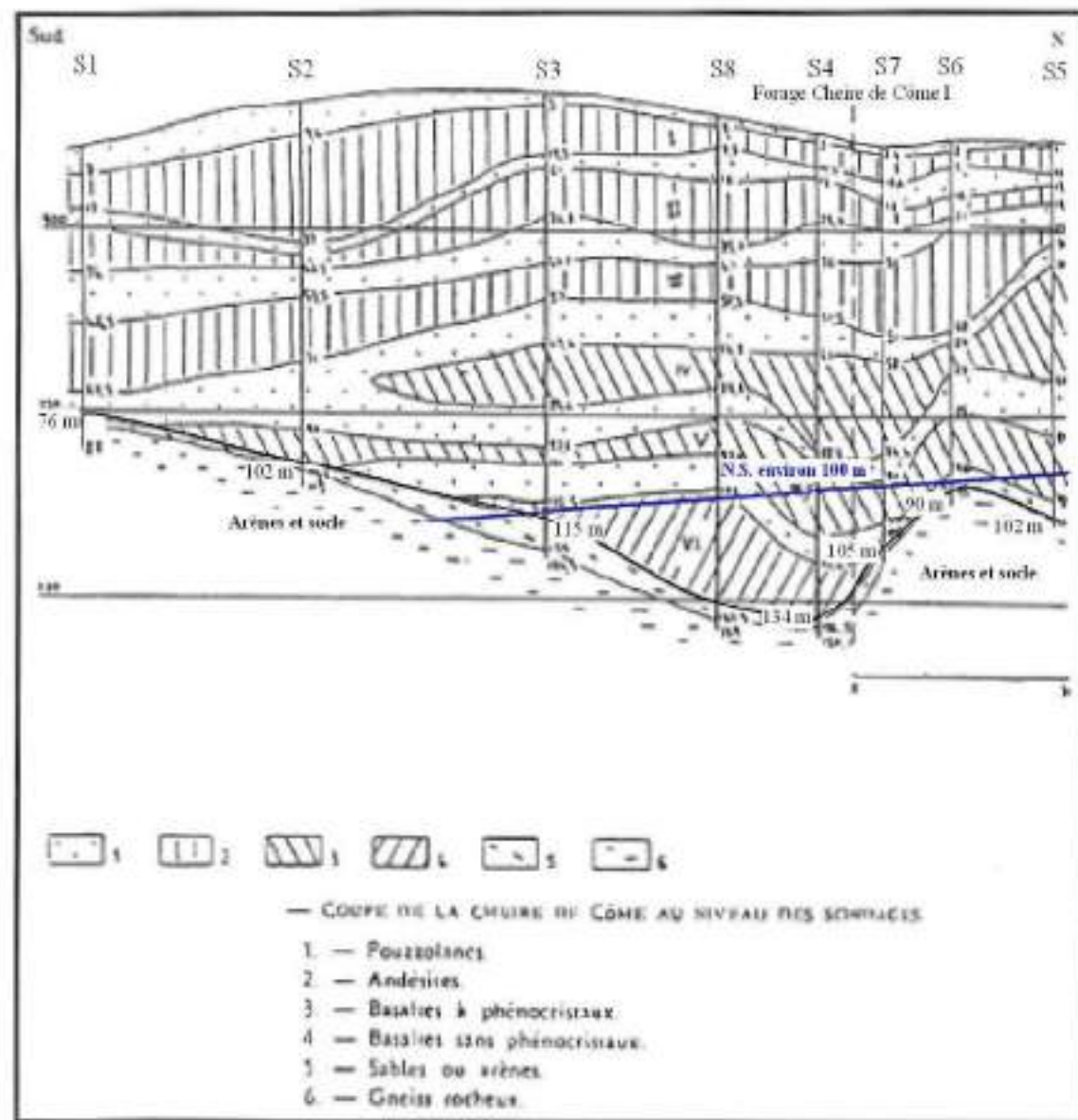
Coupe géologique Nord-Sud de la Cheire de Côme (S. Auriat, 1957)
