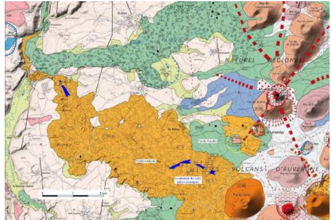
Figure 82 : Formation géologique au droit et à proximité de l'aire d'étude immédiate - Source : Carte géologique du BRGM au 1/25000
