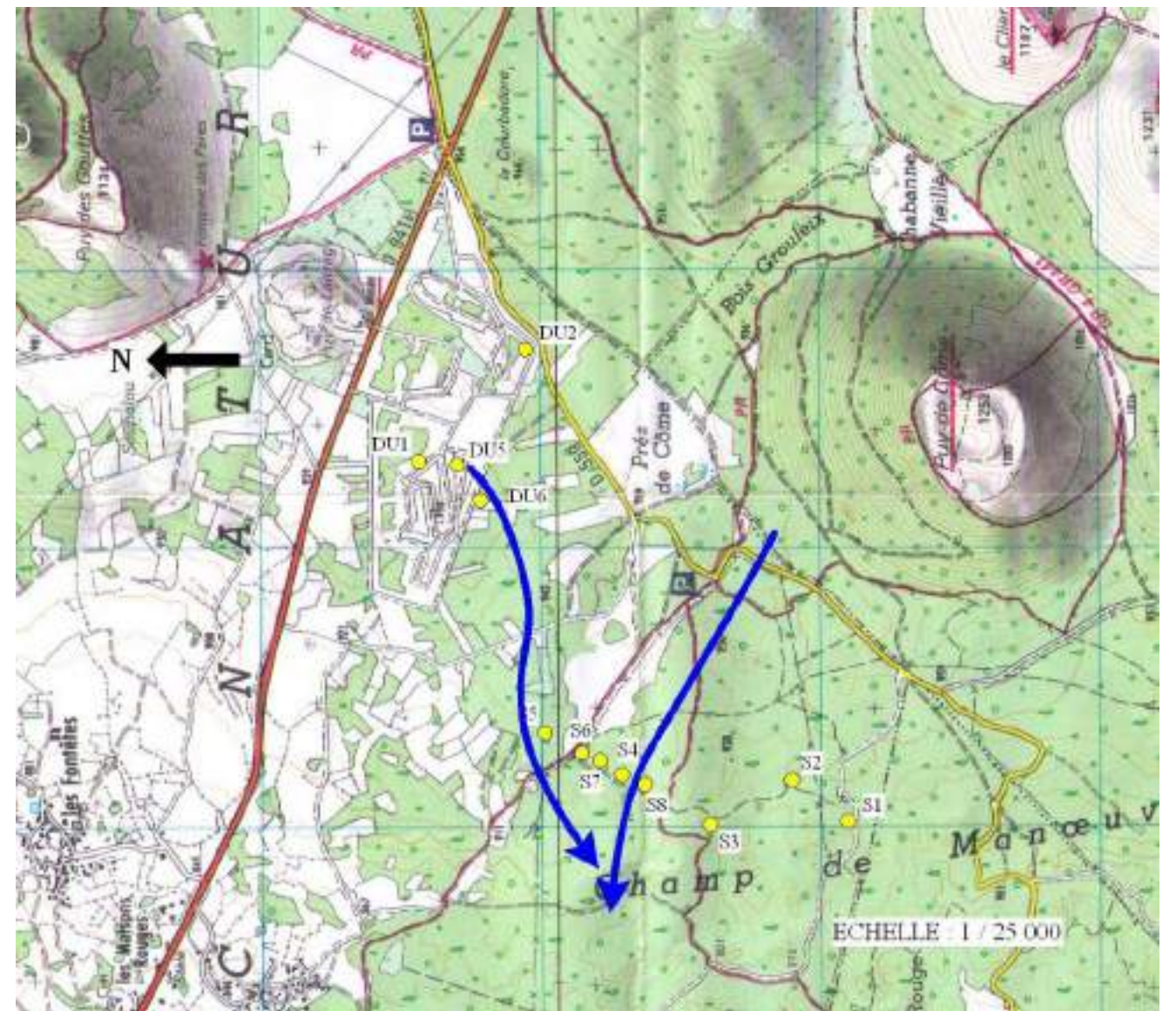
Figure 85 : Tracé revu des circulations d'eaux infra-basaltiques
