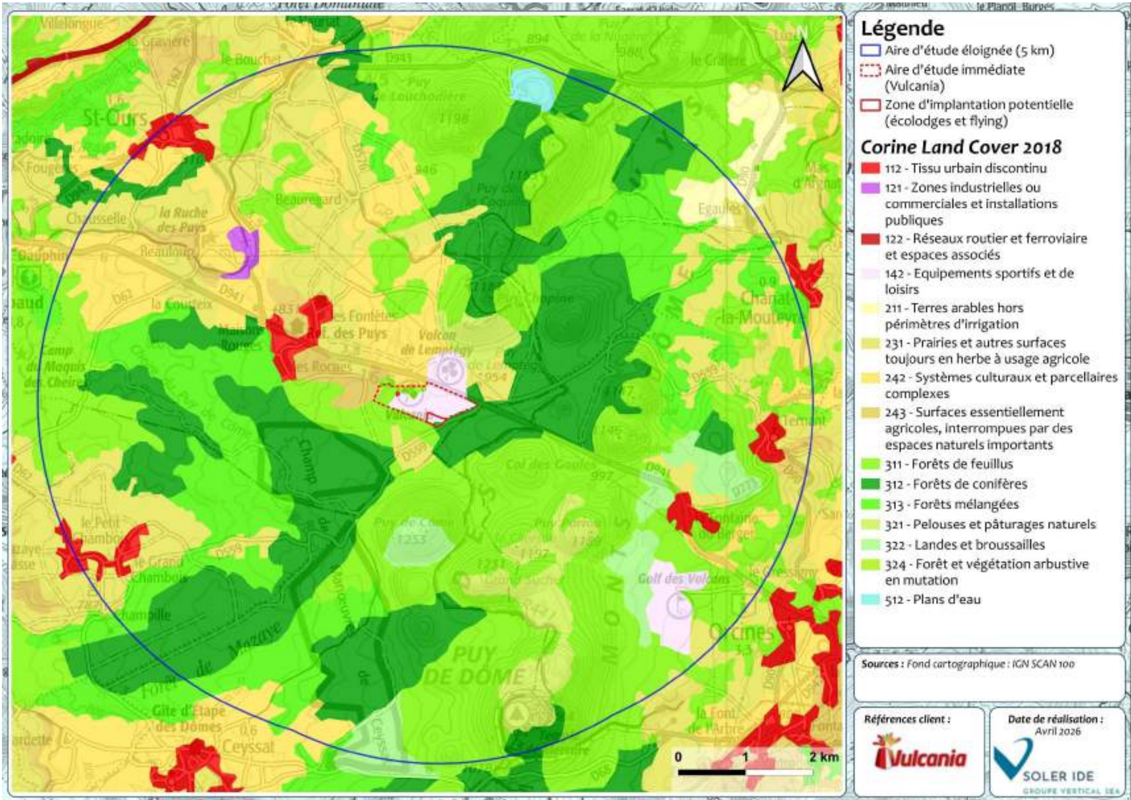
Figure 145 : Occupation du sol au droit de l'aire d'étude éloignée
