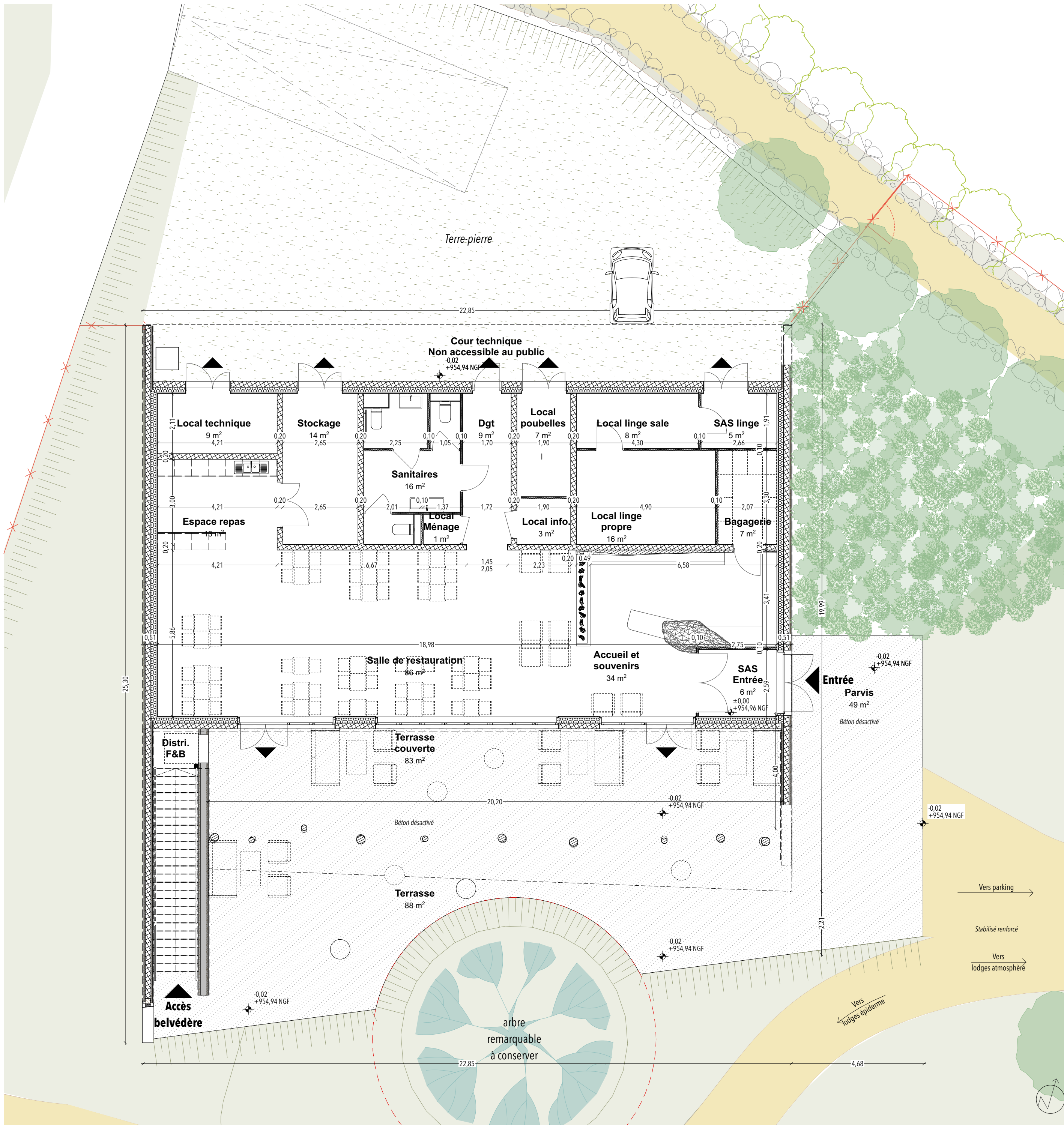
RDC ACCUEIL 1:100
