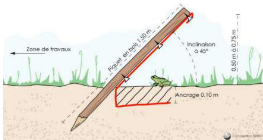
Figure 182 : Schéma d'une clôture anti-intrusion – Source : Tereo, 2014
